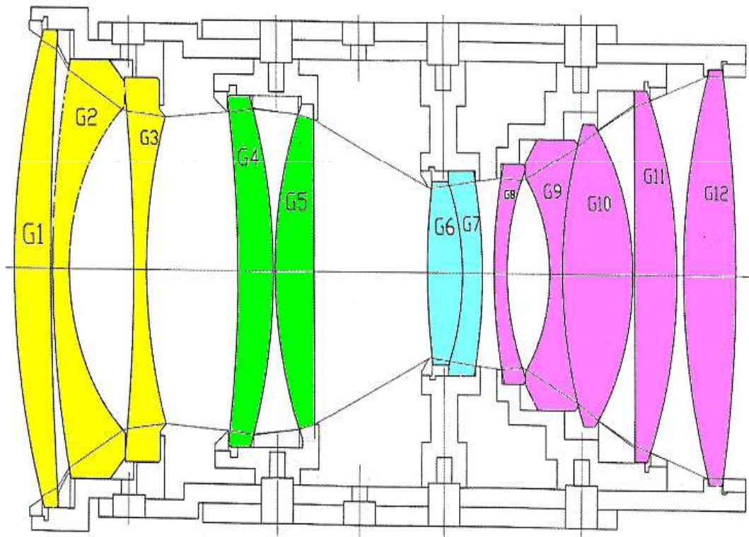
投影鏡頭構造圖
